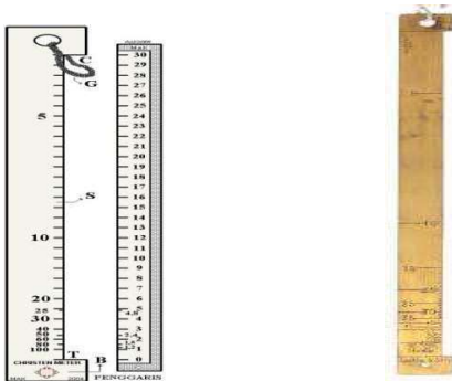
Fig. 4: Christen hypsometer
